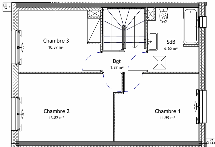
Plan de R+1
