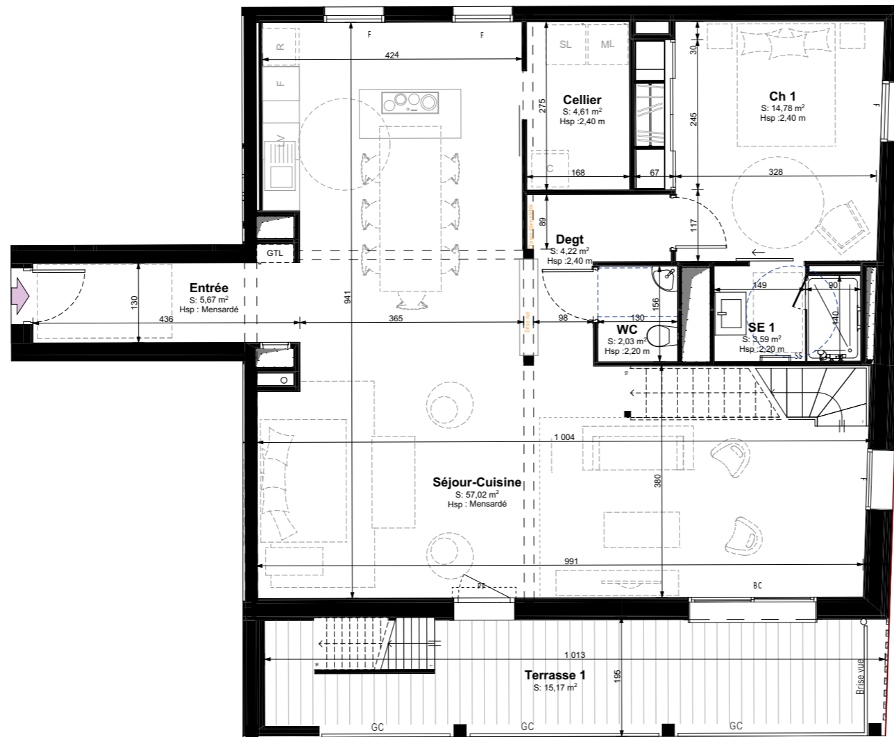
Niveau bas
