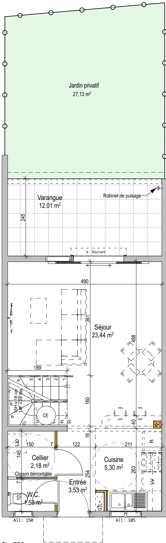
Plan RDC
