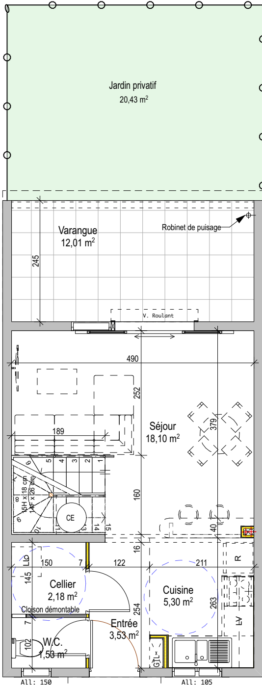
Plan RDC
