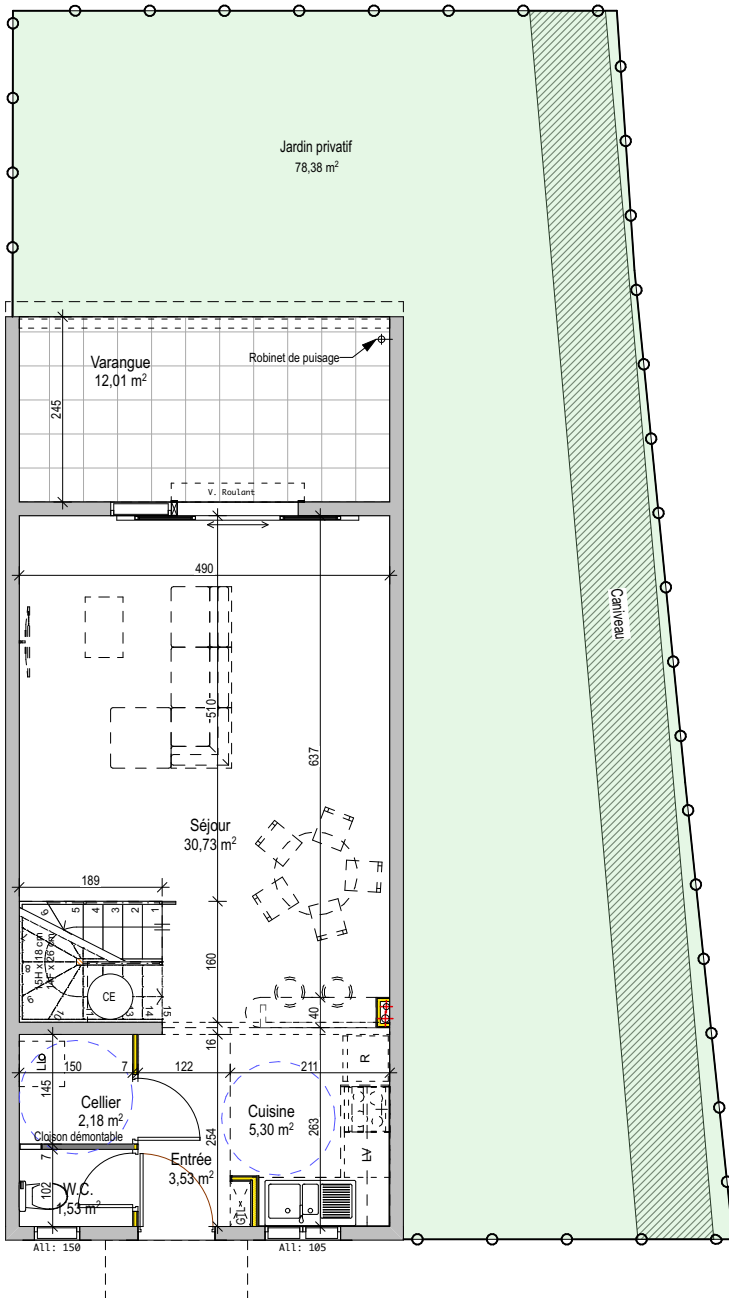
Plan RDC
