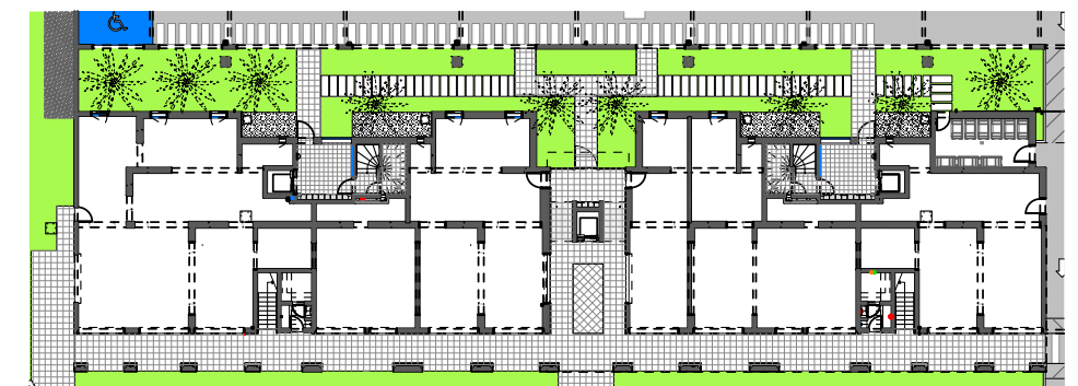
Niveau RDC (Commerce et/ou Bureau)
