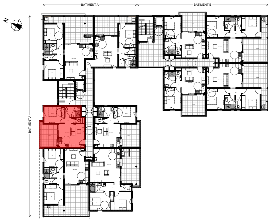
Plan de niveau - R+4 (R+3 topographique)
