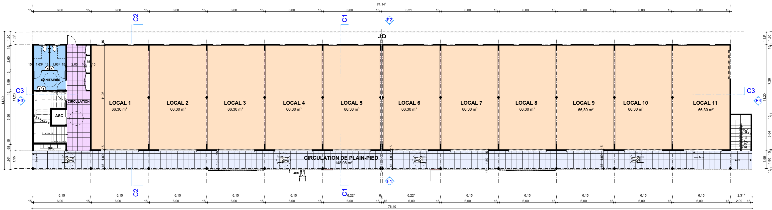
PLAN DU REZ DE CHAUSSEE SHOB : 995,30 m2
