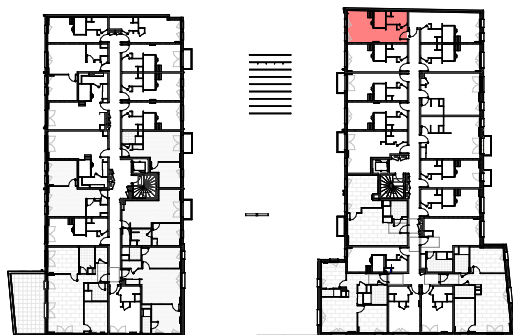
Plan de repérage appartement B-214
