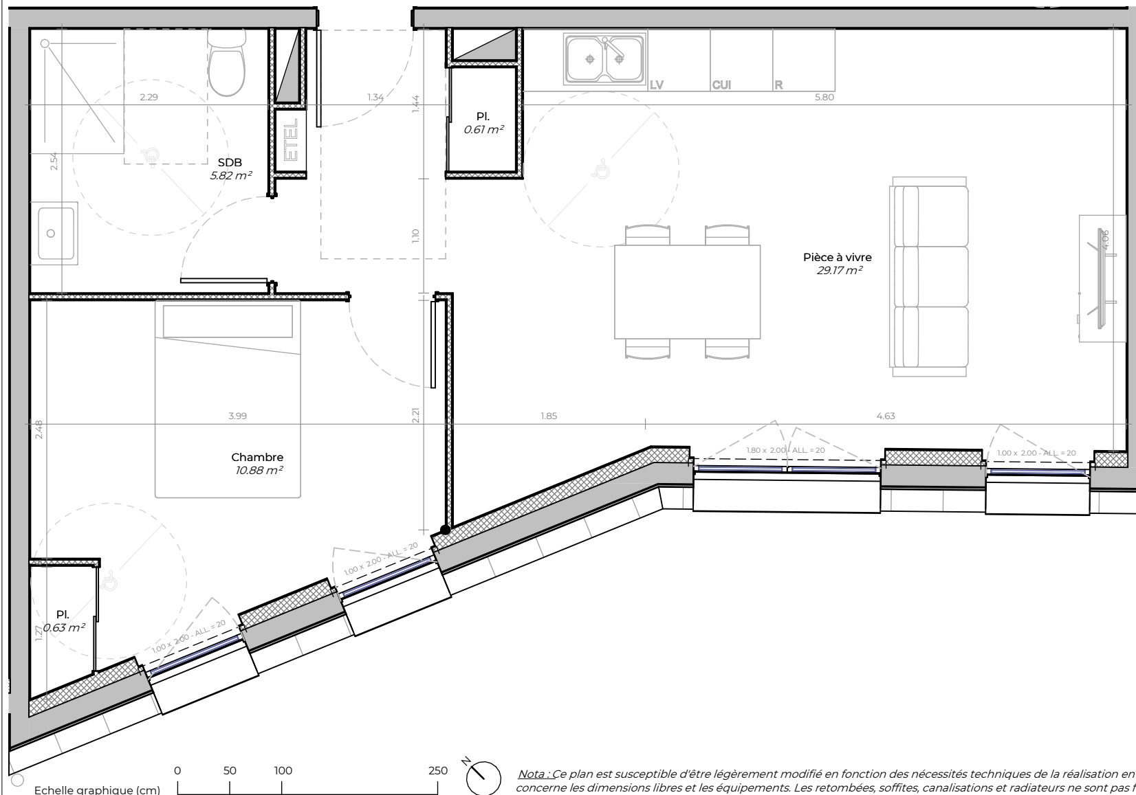
Plan de repérage: R+3
