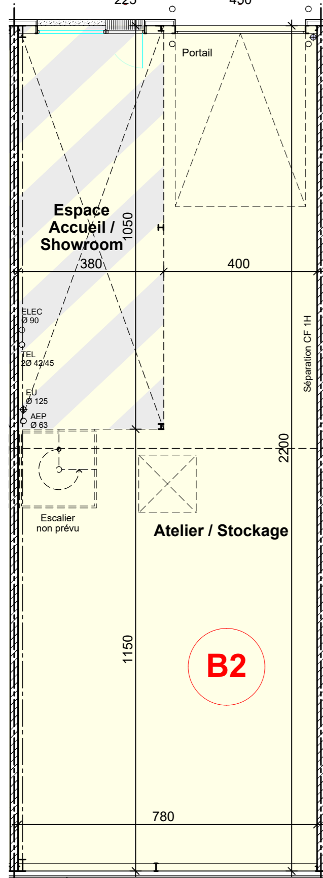
PLAN REZ-DE-CHAUSSEE
