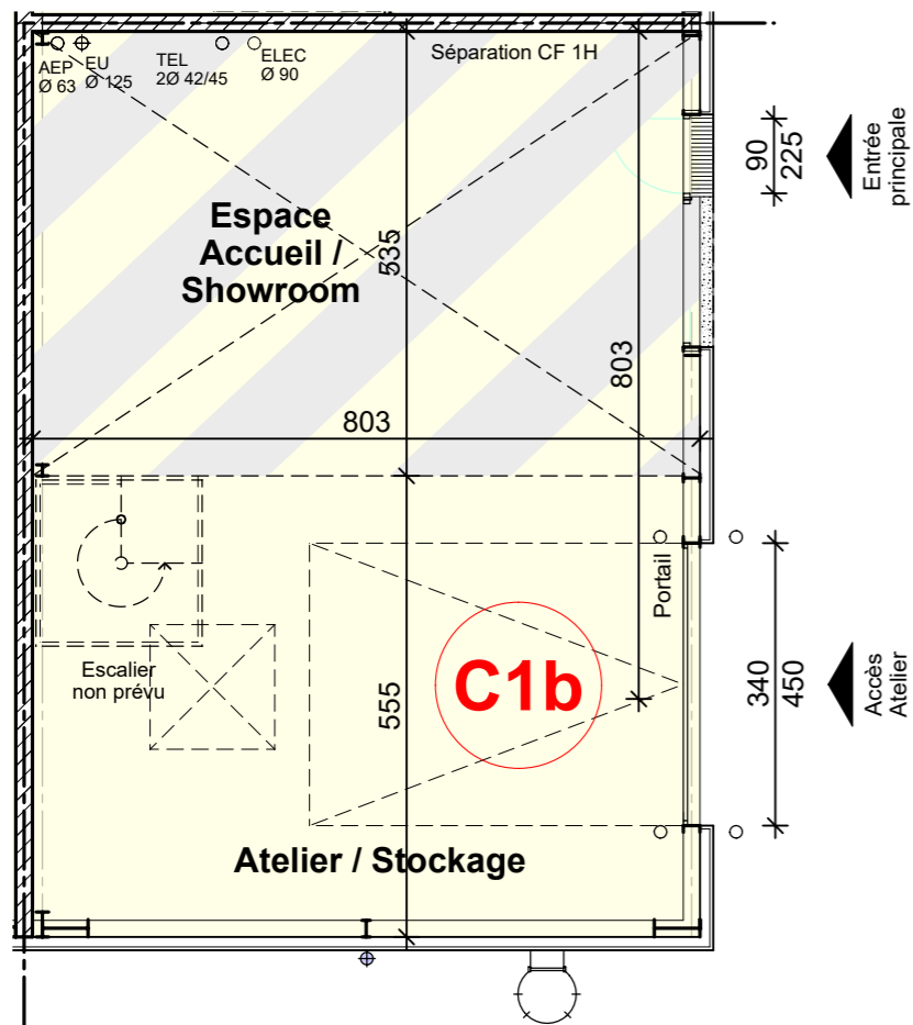
PLAN REZ-DE-CHAUSSEE
