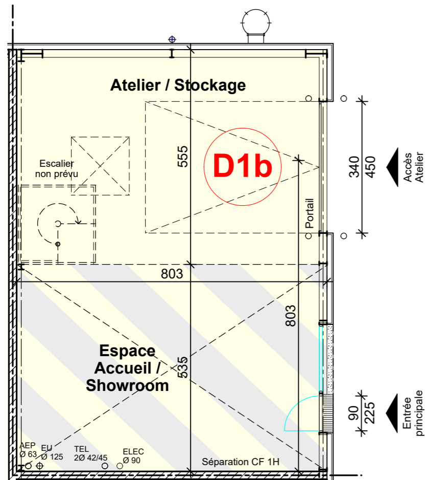
PLAN REZ-DE-CHAUSSEE
